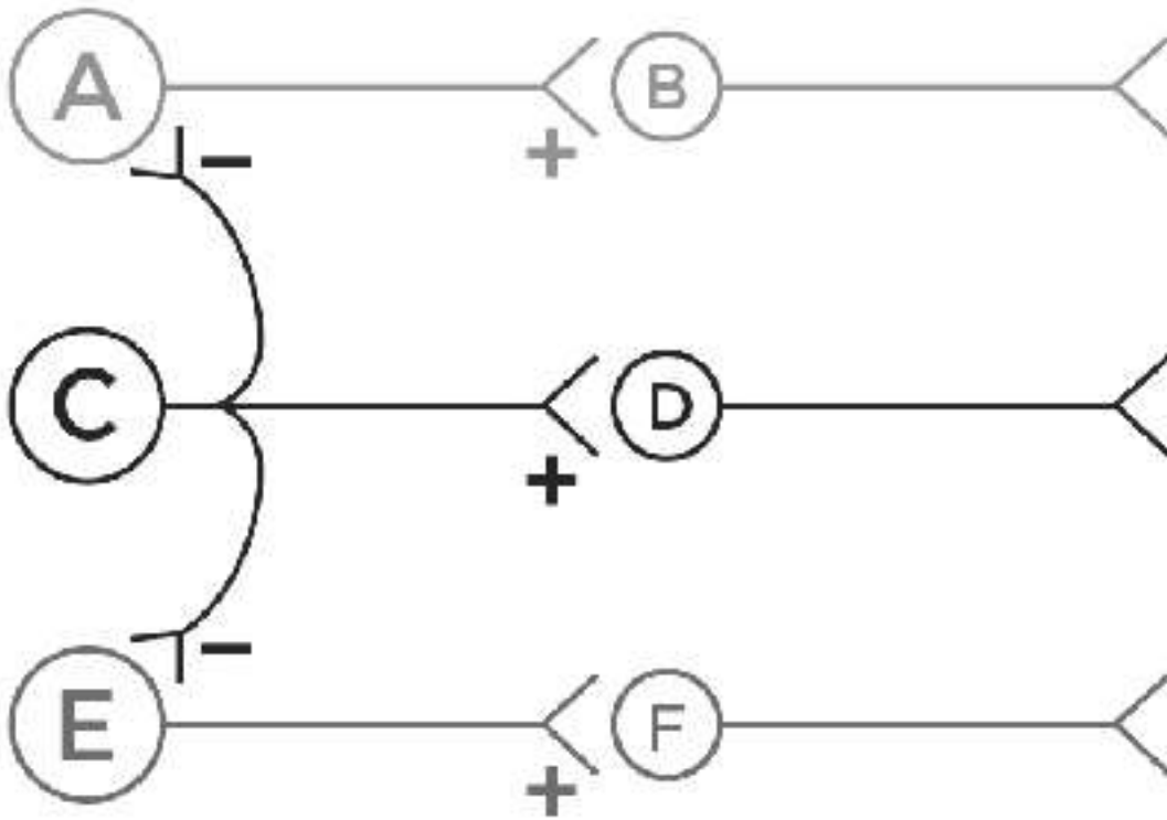
Inhibition latérale
